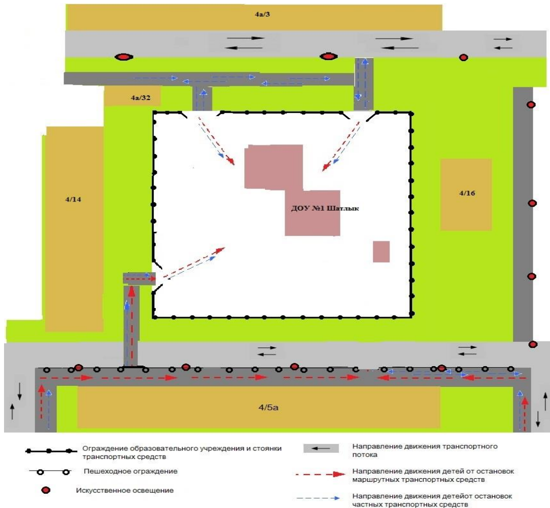
2. Схема организации дорожного движения в непосредственной близости от образовательного учреждения с размещением соответствующих технических средств организации дорожного движения, маршрутов движения детей и расположения парковочных мест
